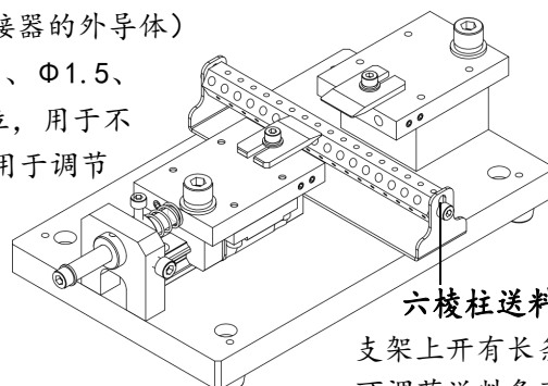
可调支架（顶面五种开孔尺寸）
