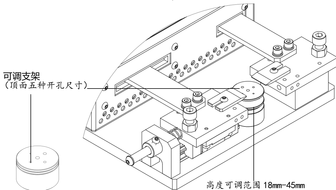
可选工装-可调支架在 ET 型焊机上的使用示意
