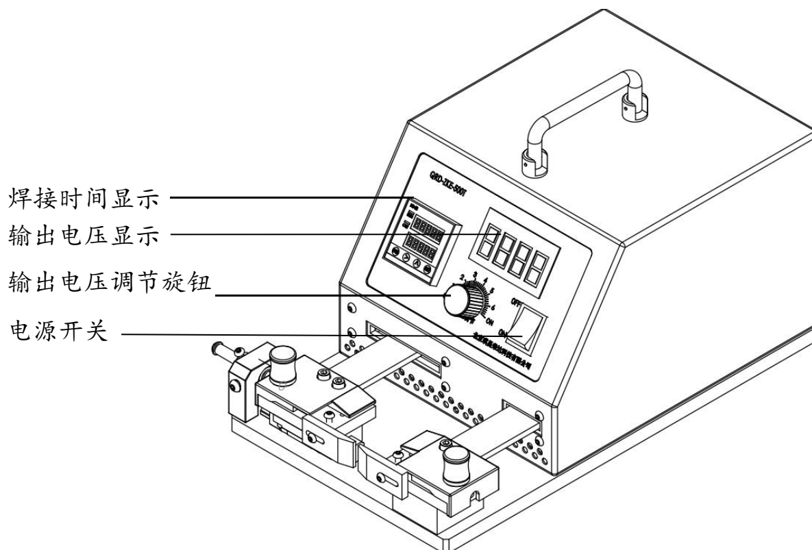
ET 型-500W 便携式精密型阻抗焊机 控制显示面板
